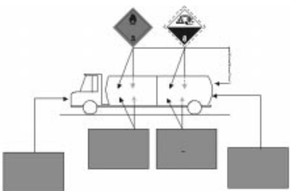
Fig. 6 Veículo Tanque compartimentado, carregado com dois ou mais produtos perigosos de classes de risco diferente, com risco subsidiário de um diferente do risco principal do outro. * - Número de Risco conforme orientação do fabricante do produto.
