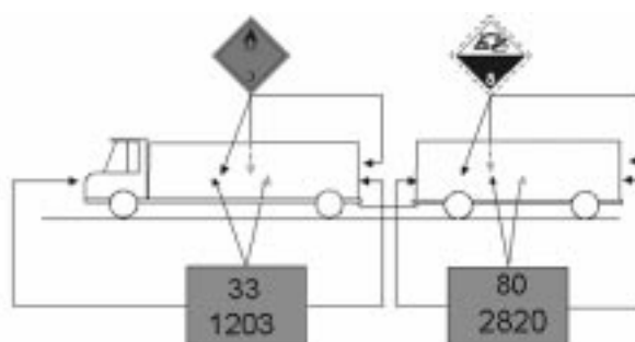
Fig. 10 Veículo de Carga Geral com um produto perigoso em quantidade igual ou inferior à quantidade isenta e vários produtos não perigosos (descartada as incompatibilidades).
