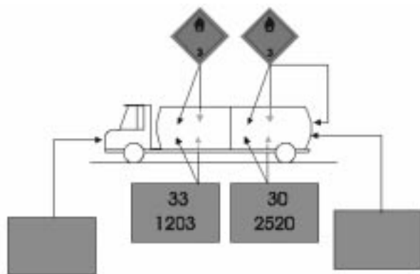
( * ) Veículo tanque com múltiplos compartimentos, carregado simultaneamente com mais de um dos seguintes produtos: álcool carburante, óleo diesel, gasolina, ou querosene, deve portar somente o painel de segurança correspondente ao produto de maior risco.
